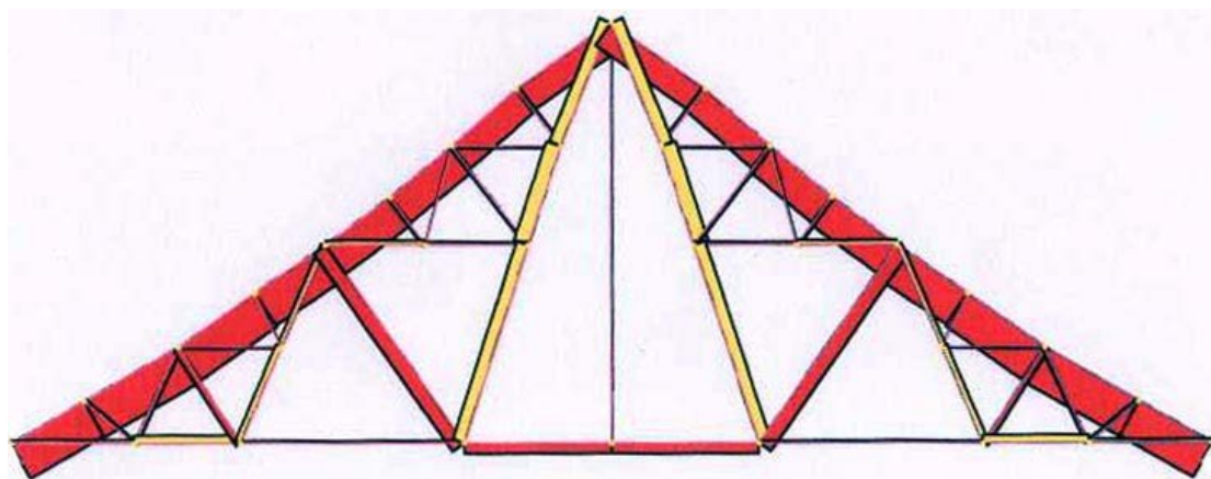
圖 3-16-3 桿件受垂直力後軸力分佈圖，色彩厚度大者代表所受力量亦較大
