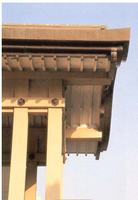
鋼筋混凝土樑柱仿木構件 錄自傅朝卿 1995《臺南市日據時代歷史性建築》 P.205
