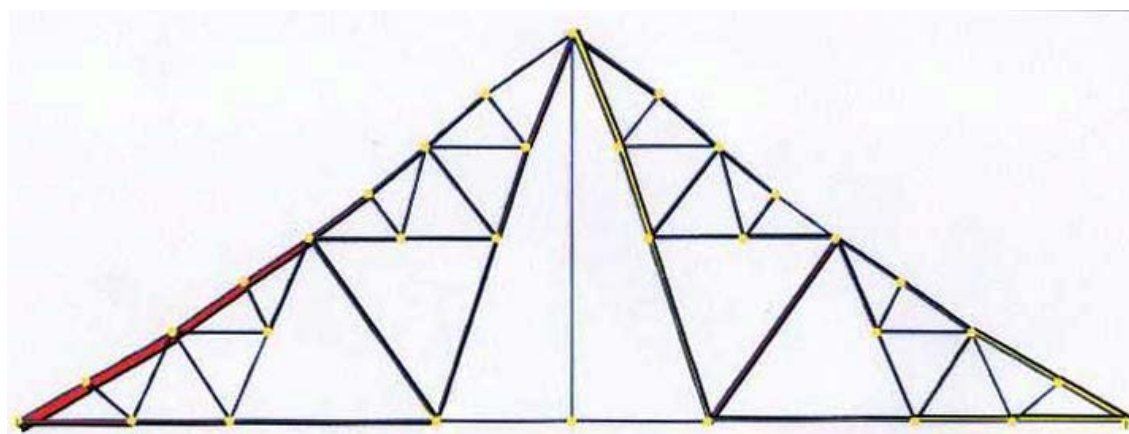
圖 3-16-5 桿件受水平力後軸力分佈圖，色彩厚度大者代表所受力量亦較大
