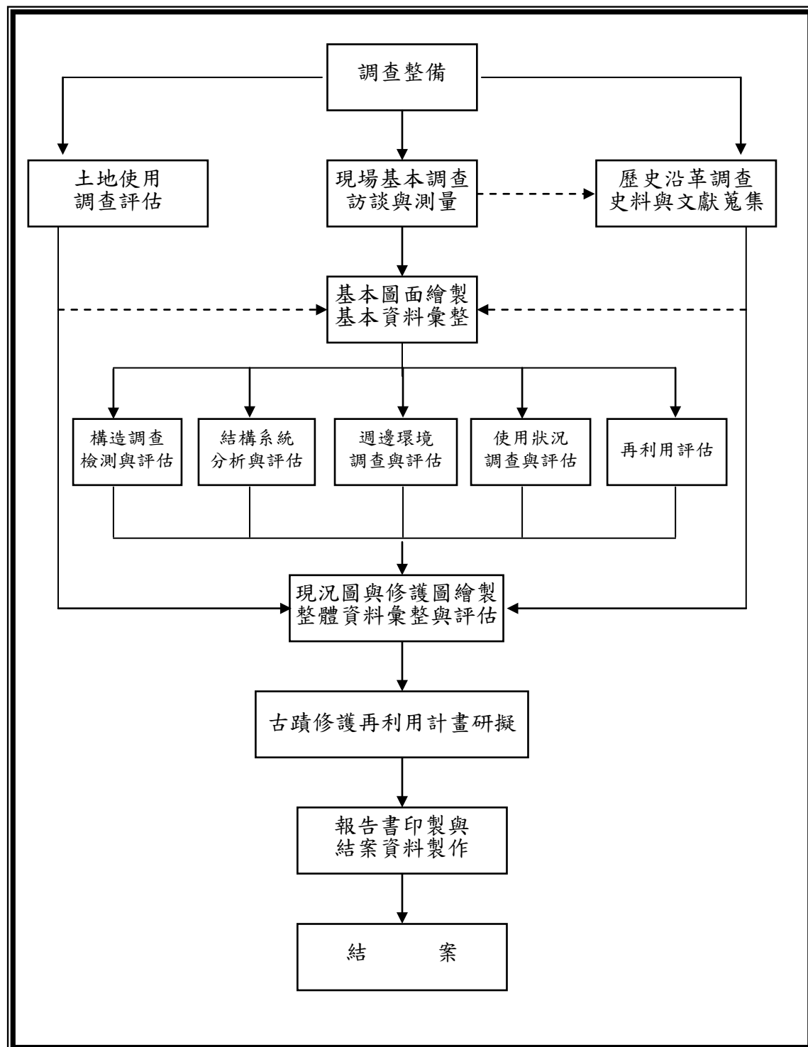
圖 1-2-1 研究流程圖
