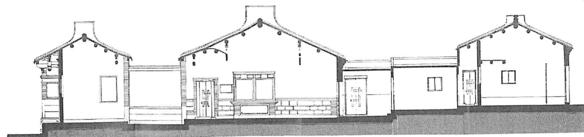
右邊架縱剖面圖
