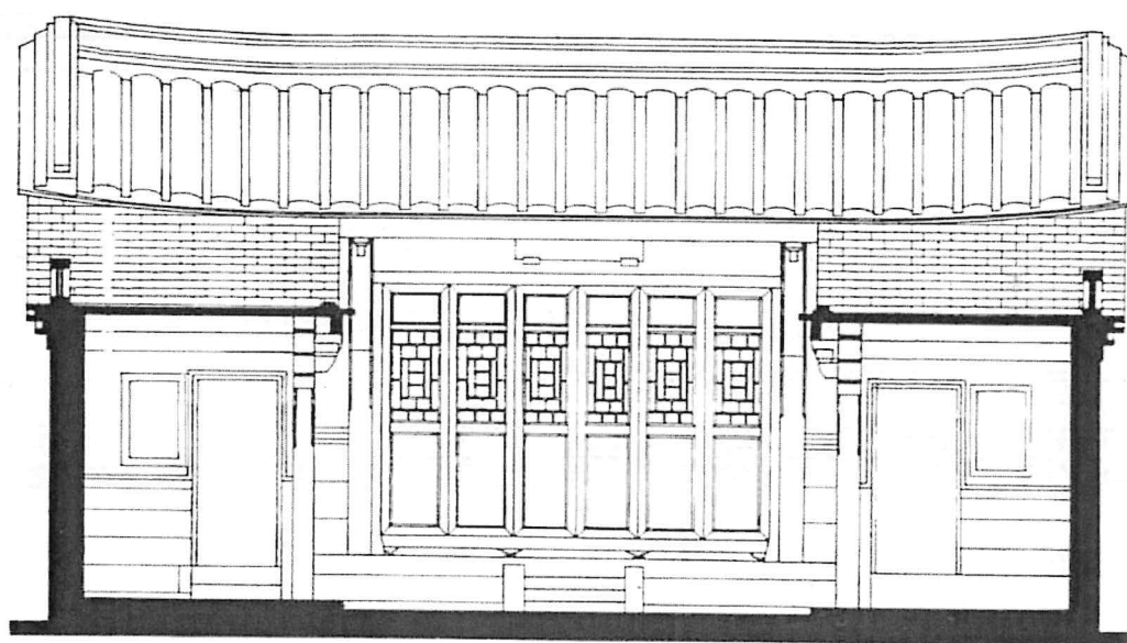
後殿正立面圖
