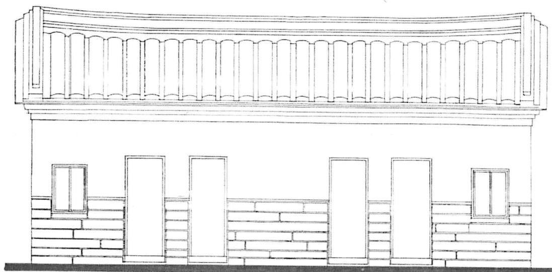
後殿背立面圖
