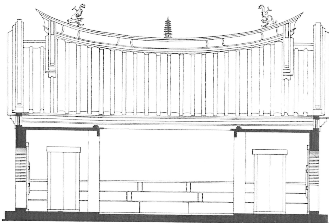
正殿背立面圖（含左右迴廊剖面）
