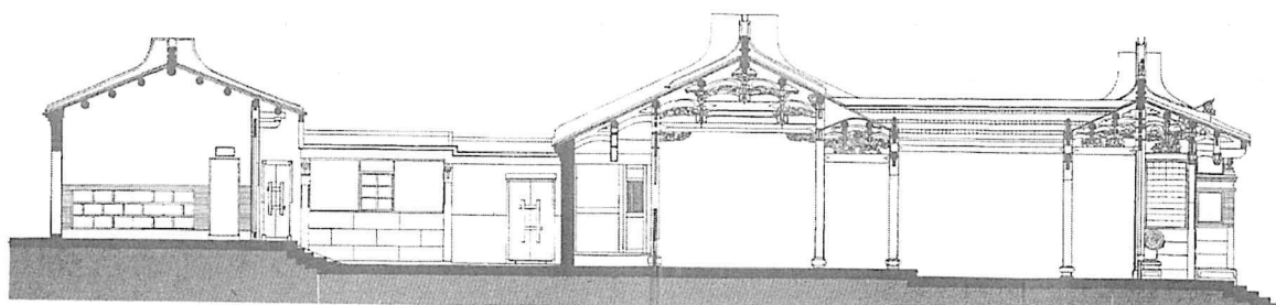
明間縱剖面圖(左架)
