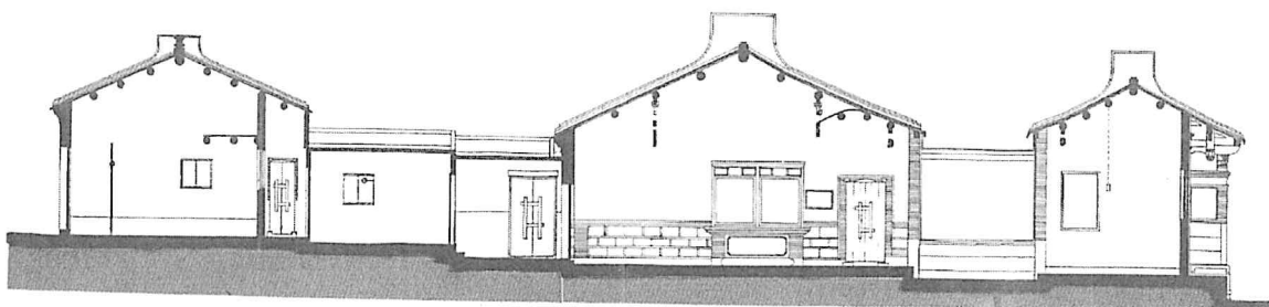
左邊架縱剖面圖
