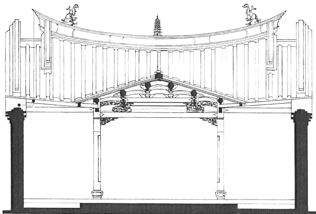
正殿正立面圖
