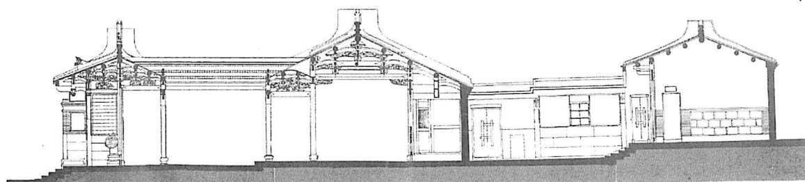
明間縱剖面圖(右架)
