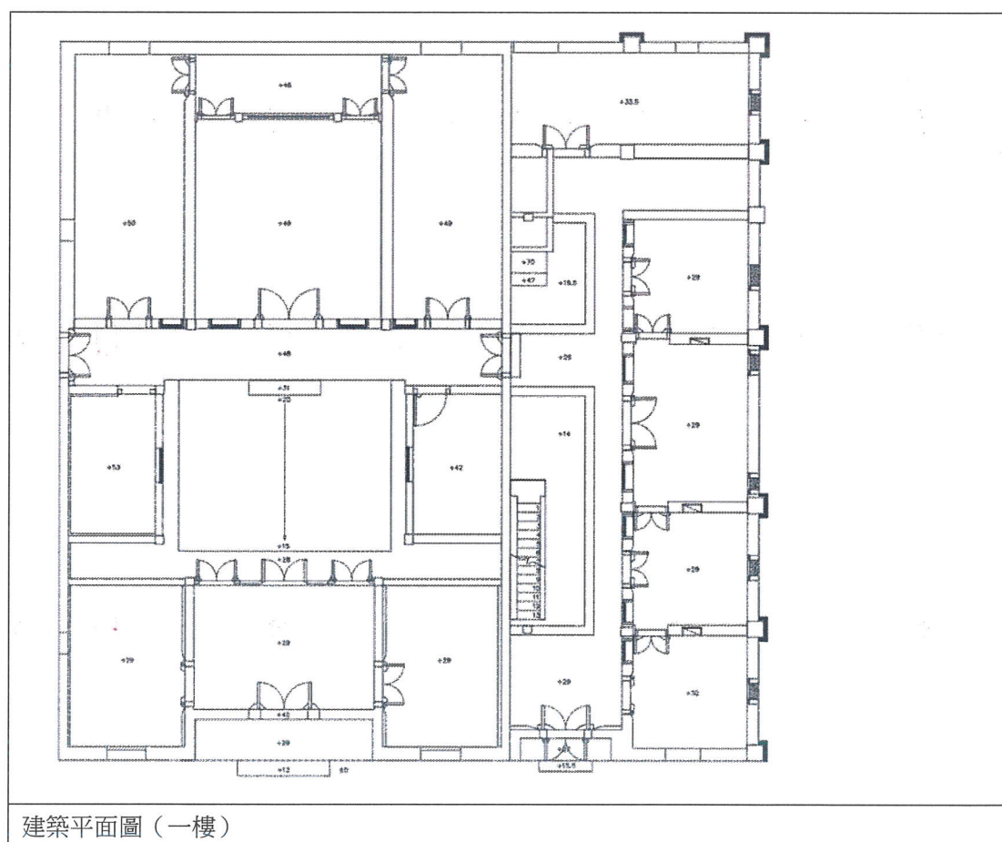
地籍圖套繪建築平面圖
