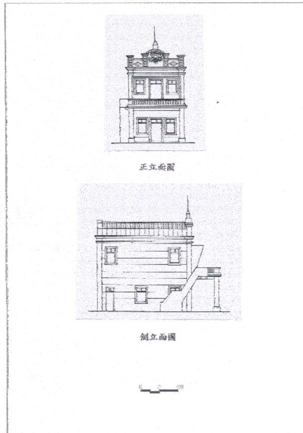
鹽田鹽務辦公室立面圖
