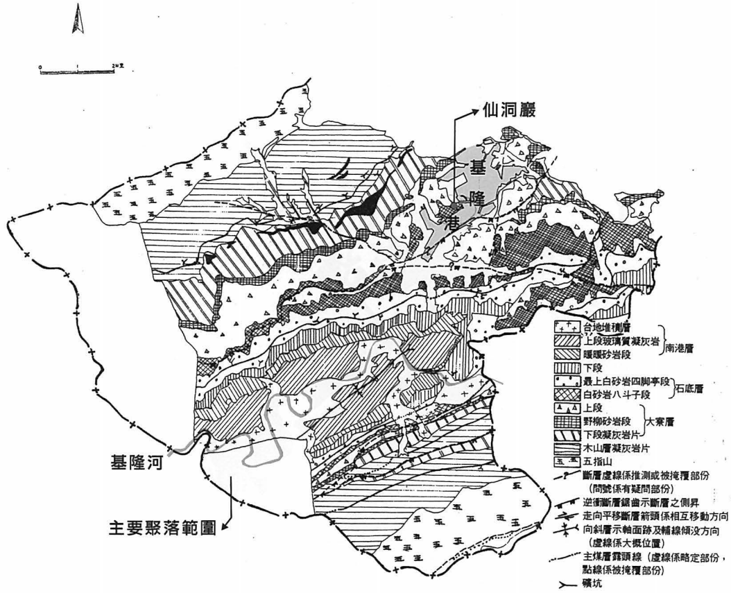
圖 2-2 基隆市地質分類圖（基隆市都市計畫年報與本研究整理）
